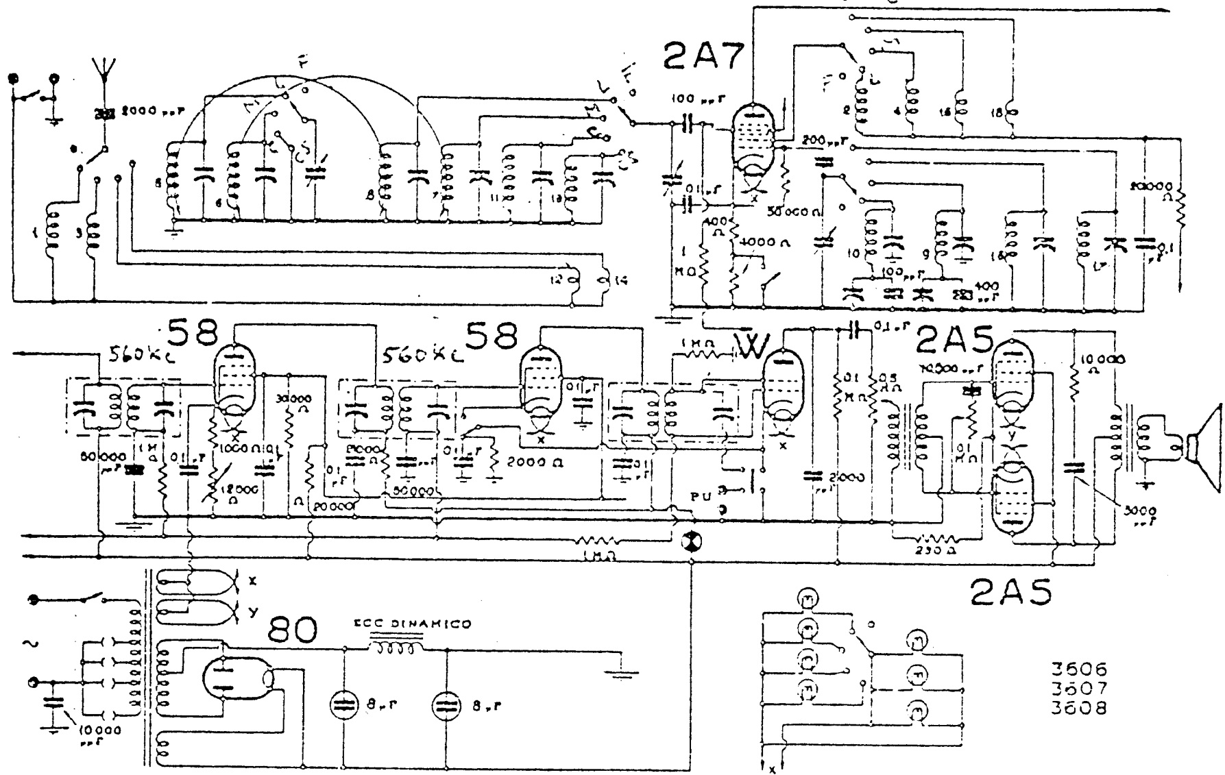
UNDA RADIO - MODD. « TRI UNDA 7 » « 77 » « 77c »
